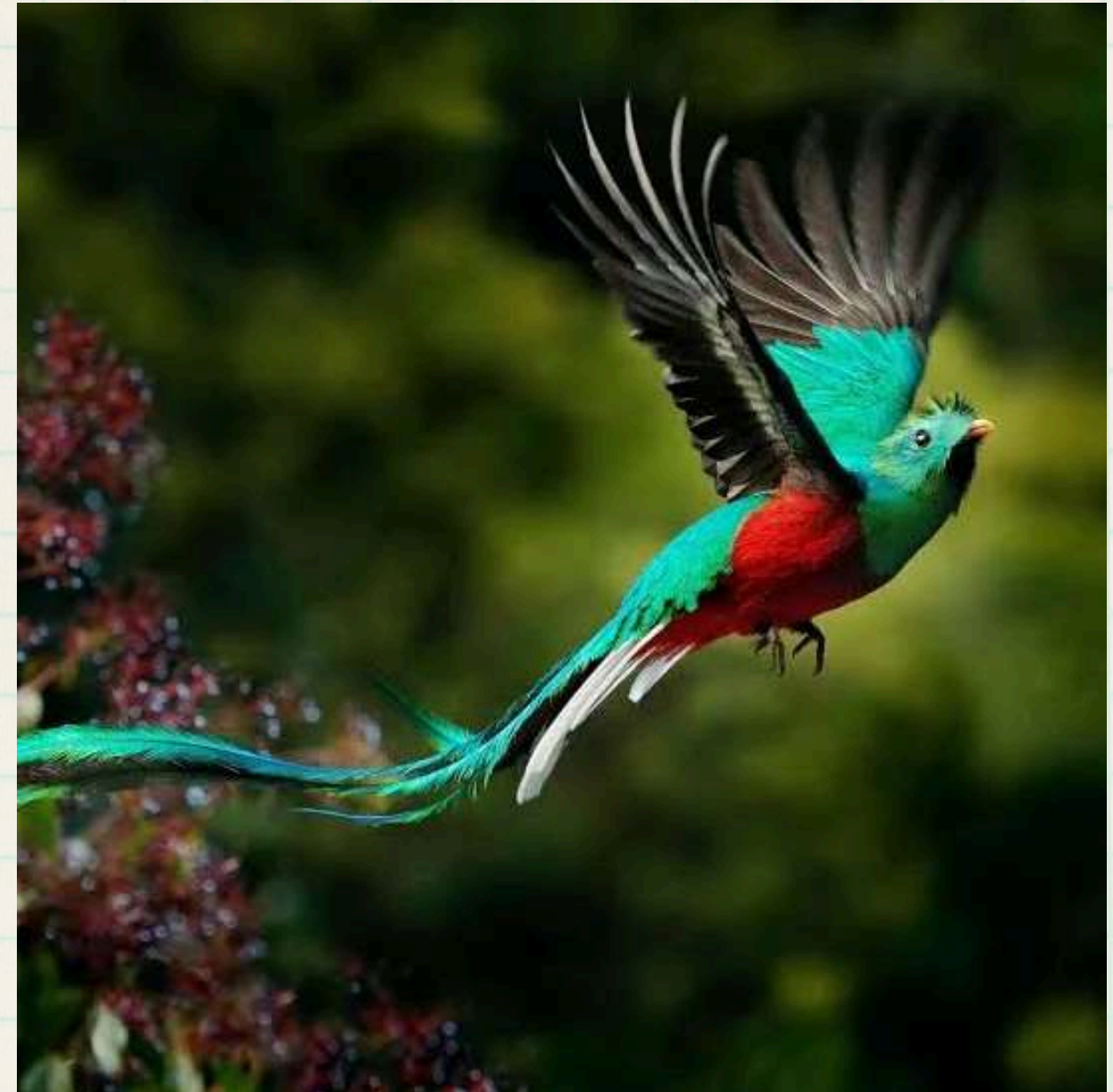
QUETZAL
